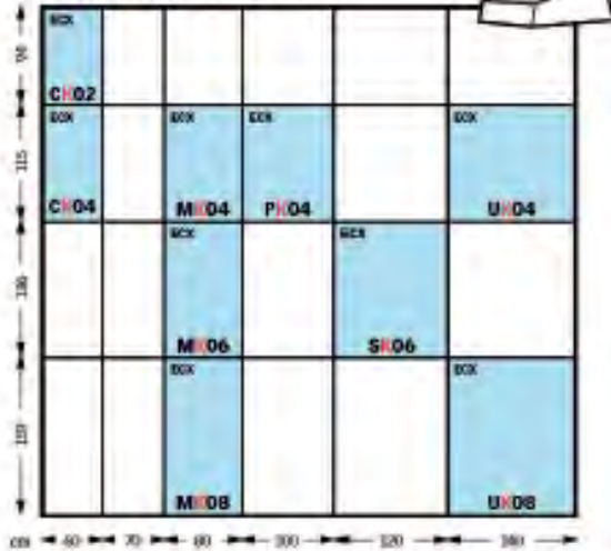
Raccordi per tetti piani con griglia
